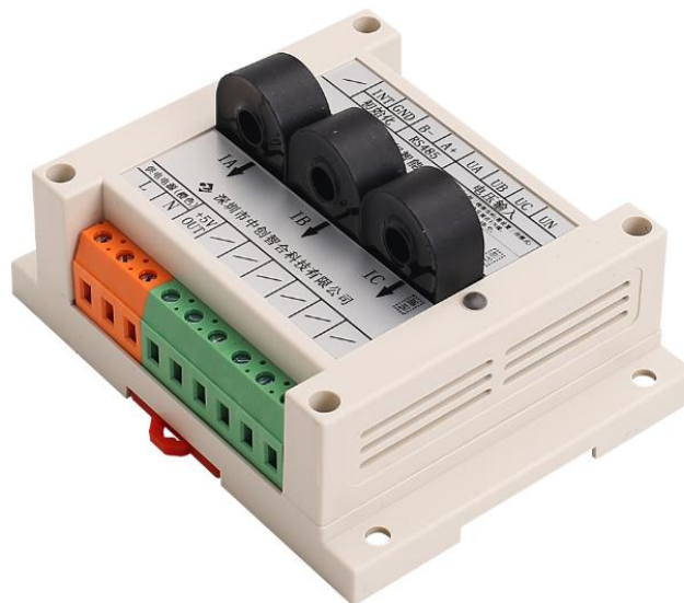
图 4.2、电流穿孔输入外观图（孔径 7.5mm）
