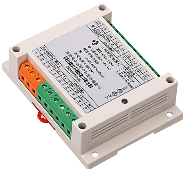
图 4.1、电流端子输入外观图（导轨安装）
